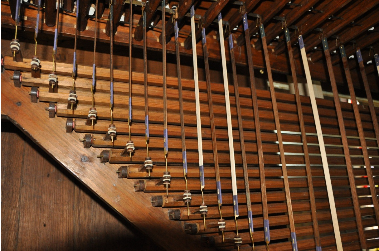
Wiedereinbau der restaurierten technischen Anlage (hier: Wellenbrett der mechanischen Spieltraktur)
